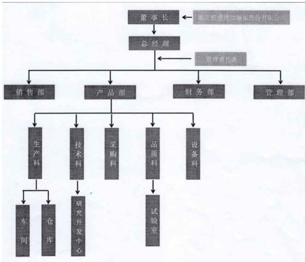
图 3.2 组织机构图
